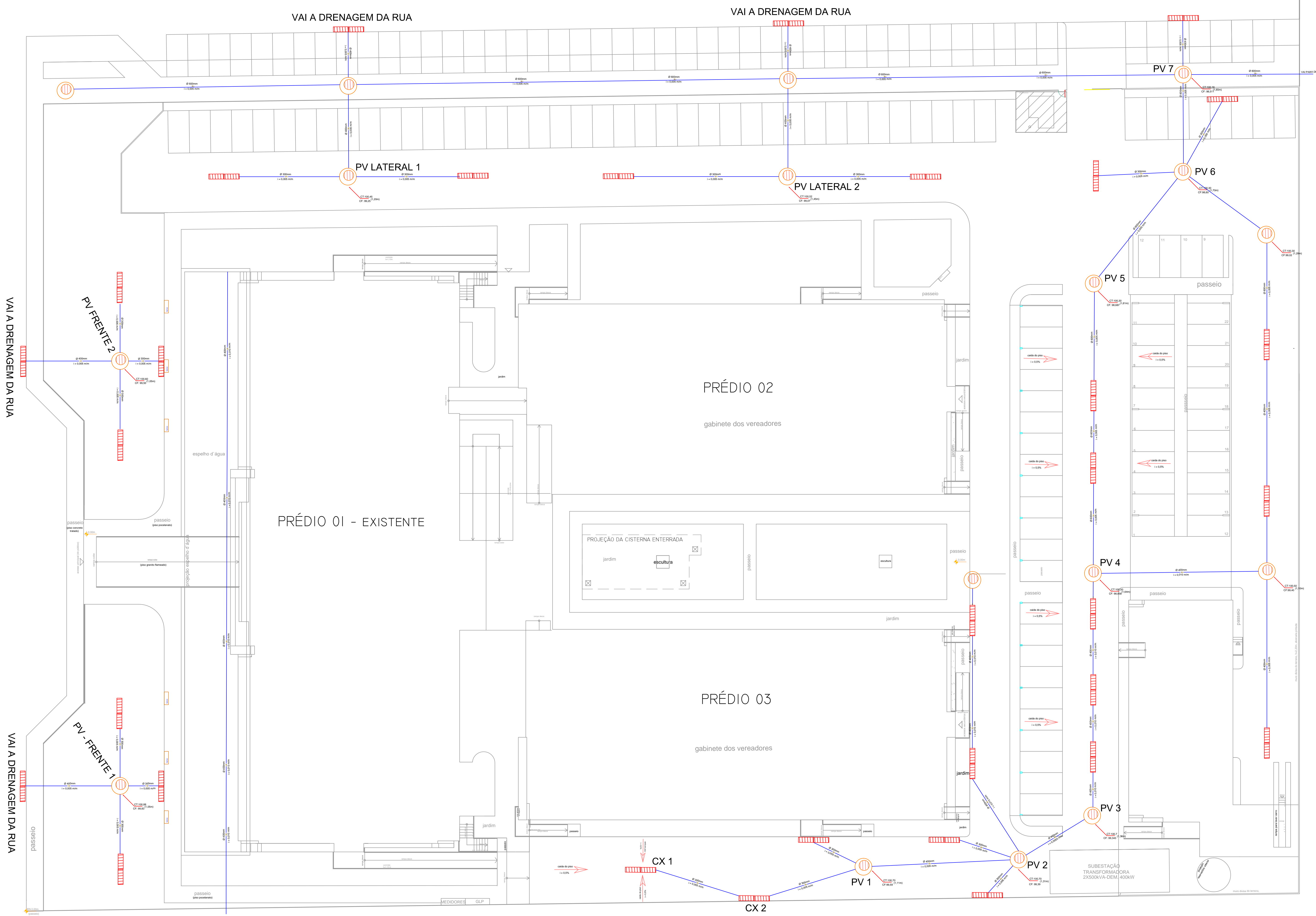
PLANTA BAIXA - DRENAGEM ESC. 1:200
