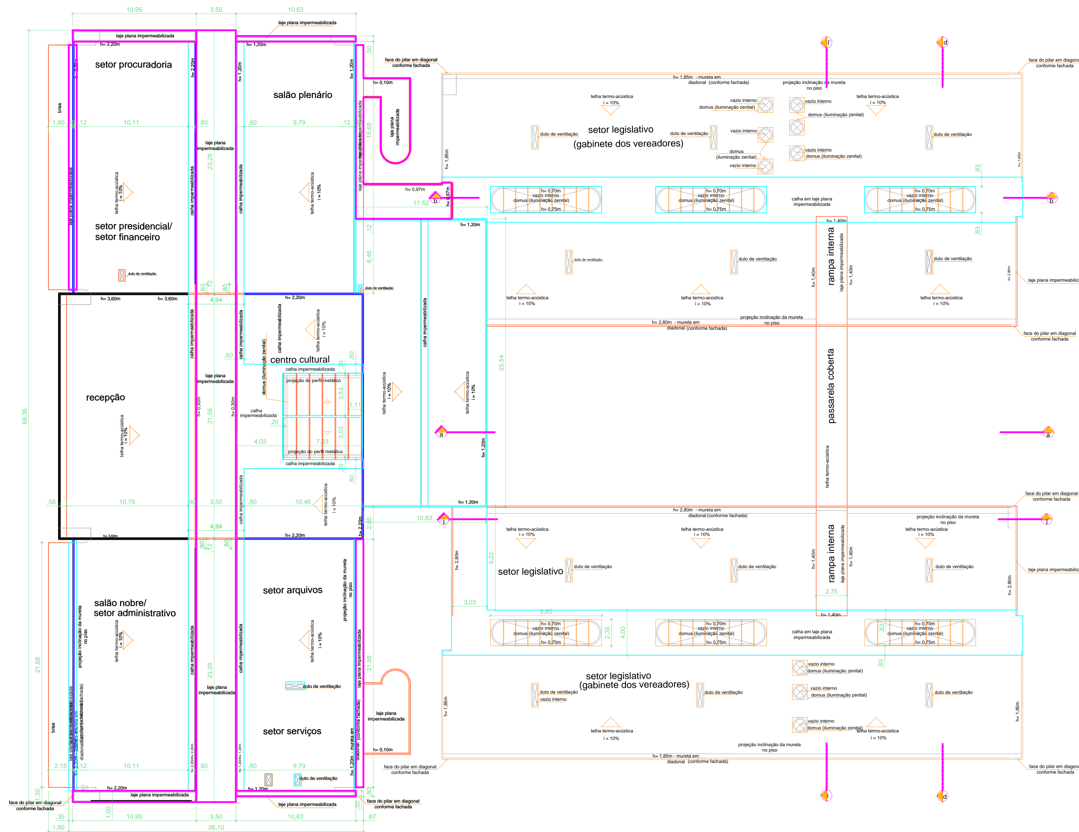
DIAGRAMA COBERTURA CÂMARA escala 1/200
